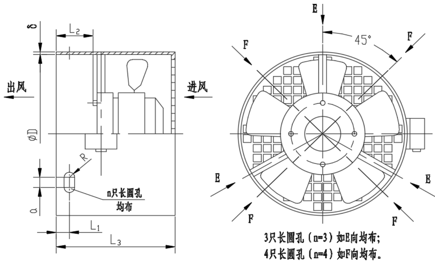
G 系列 YVP 变频调速电机风机
